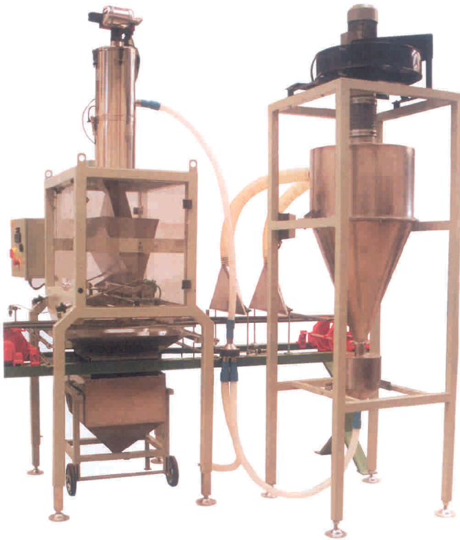
Equipo aspiradora y granilladora Vacuum and granule application units Equipe d'aspiration et granule
