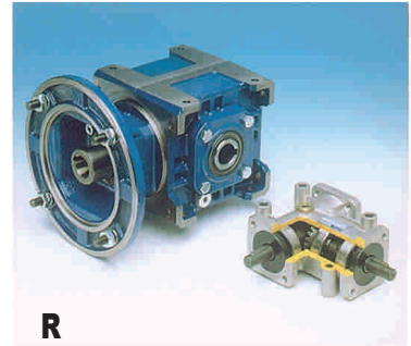
Rinvii angolari Right angle gearboxes Winkelgetriebes
