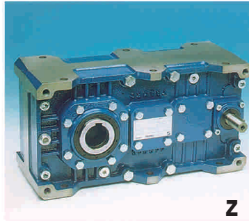
Riduttori ad assi paralleli Parallel gear shaft units Getriebe mit parallele achsen
